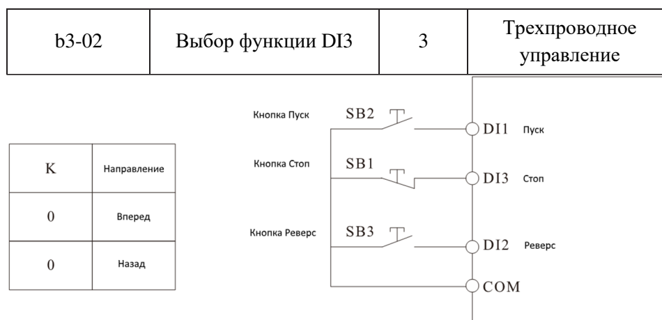
Рис. 5-13 Настройка трехпроводного режима 2
