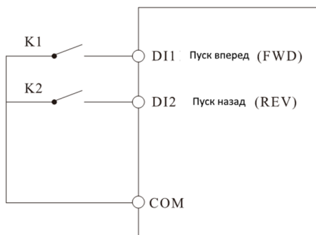
Рис. 5-10 Настройка двухпроводного режима 1
