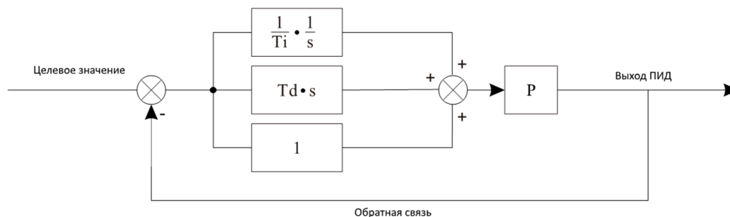
Рис. 6-25 Блок-схема ПИД-регулирования.
