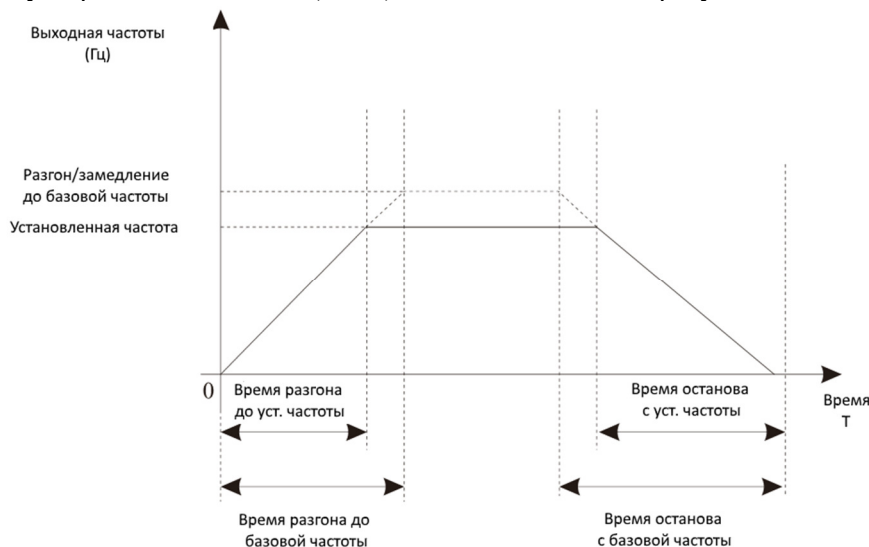
Рис. 5-3 Время разгона/торможения
