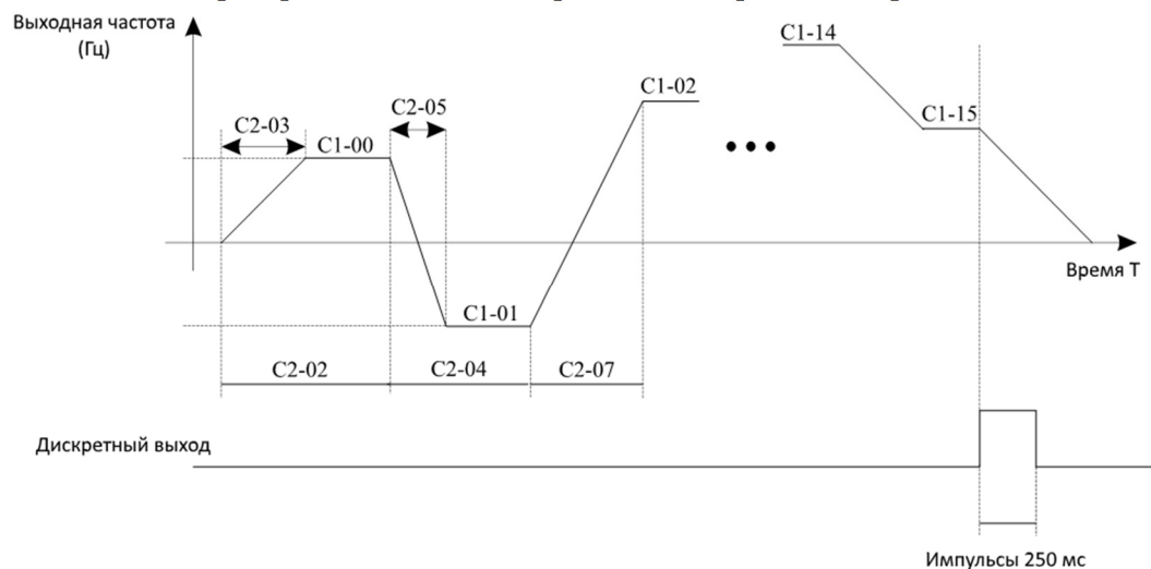
Диаграмма 5-28 Использование ПЛК в качестве источника частоты
