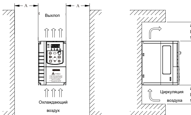
Рис. 3-1 Обеспечение вентиляции на месте установки
