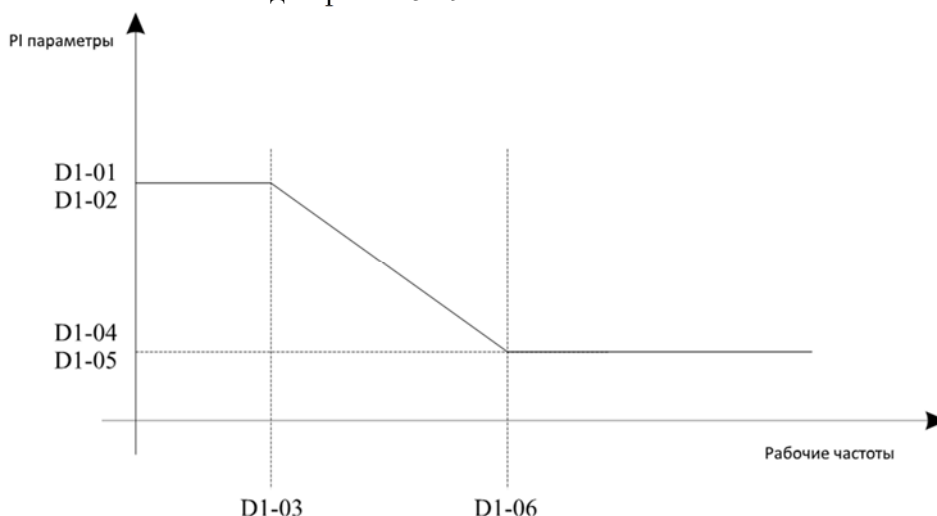
Диаграмма 5-29. Связь между рабочими частотами и параметрами PI
