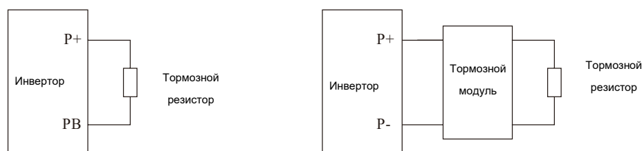
Рис. 2-10 Подключение тормозного модуля и резистора
