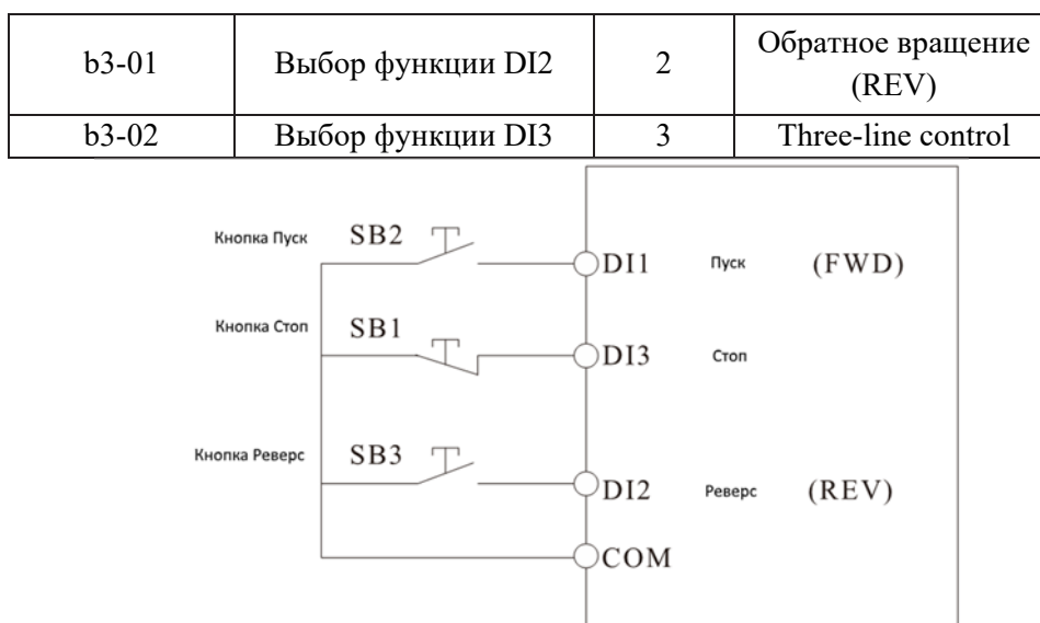
Рис. 5-12 Настройка трехпроводного режима 1
