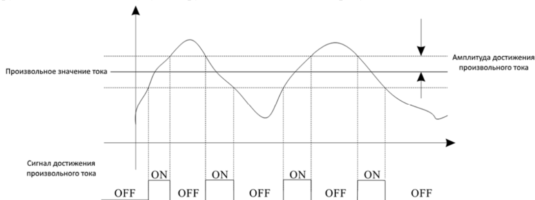
Рис. 5-19 Обнаружение достигнутого тока
