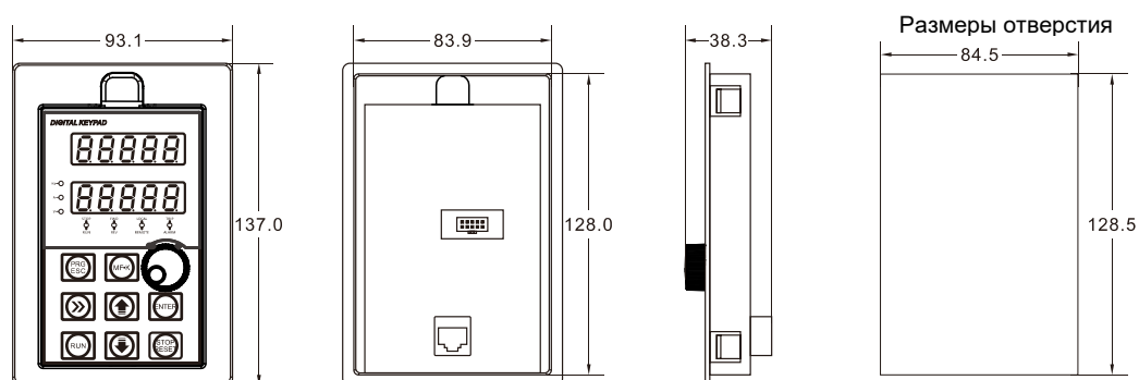
Рис 2-9 Внешний вид и размеры съемной панели преобразователей большой мощности
