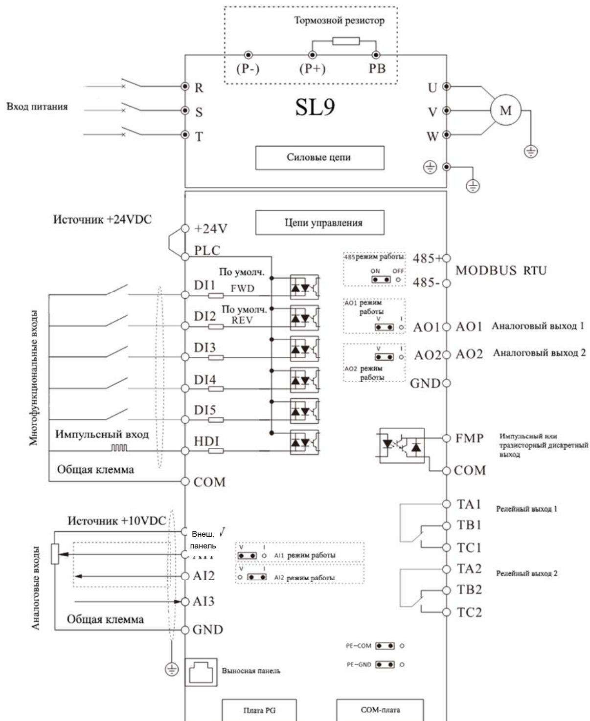
Рис. 3-11 Схема цепей управления и силовых цепей
