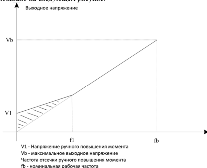
Диаграмма 5-30 Ручное повышение крутящего момента
