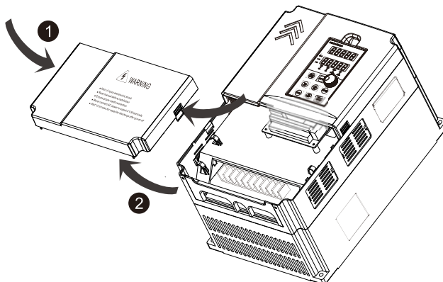
Рис. 3-5 Снятие крышки пластикового корпуса
