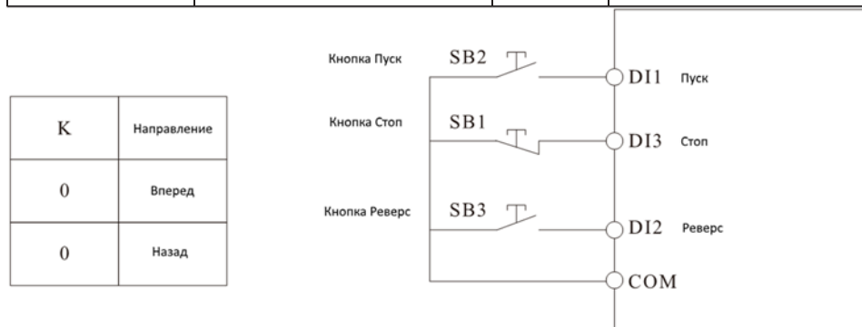
Рис. 5-13 Настройка трехпроводного режима 2
