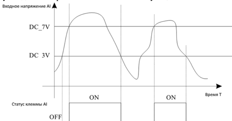
Рис. 5-22 Взаимосвязь входного напряжения AI и соответствующего состояния DI
