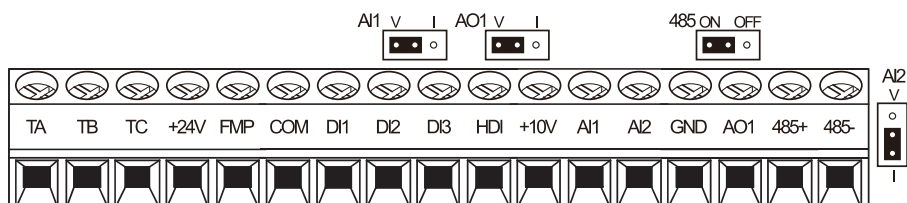
Рис 3-13 Преобразователи вход 1х220, выход 3х0...220В, 2,2кВт, вход 1х220, выход 3х0...380В, 2,2-4кВт, вход 3х380, выход 3х0...380В, 4-5,5кВт
