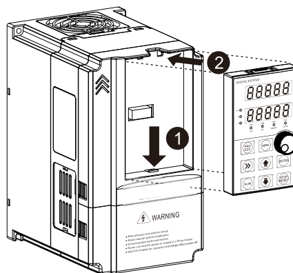
Рис. 3-3 Удаление панели управления (клавиатуры) Рис. 3-4 Установка панели управления (клавиатуры)
