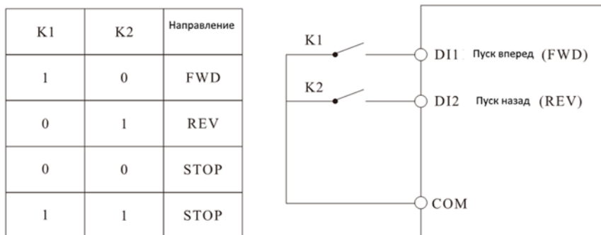
Рис. 5-10 Настройка двухпроводного режима 1
