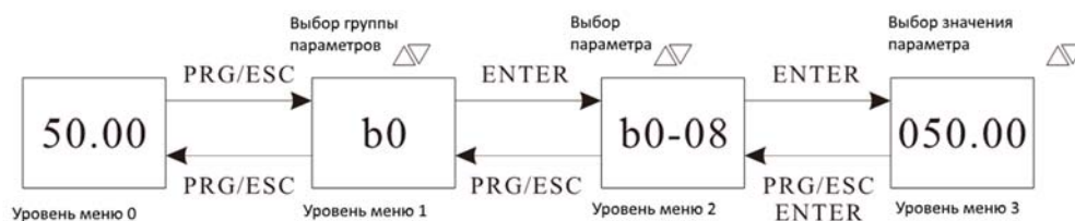
Рис. 4-2 Порядок работы с панелью управления
