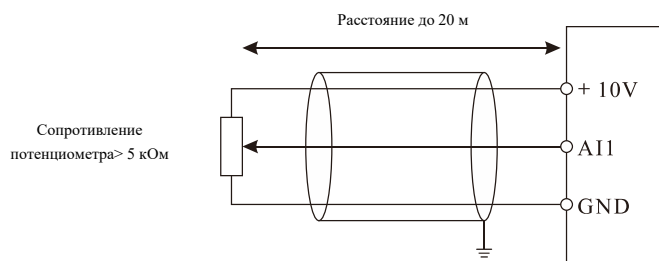
Рис. 3-15 Подключение аналоговых входных клемм
