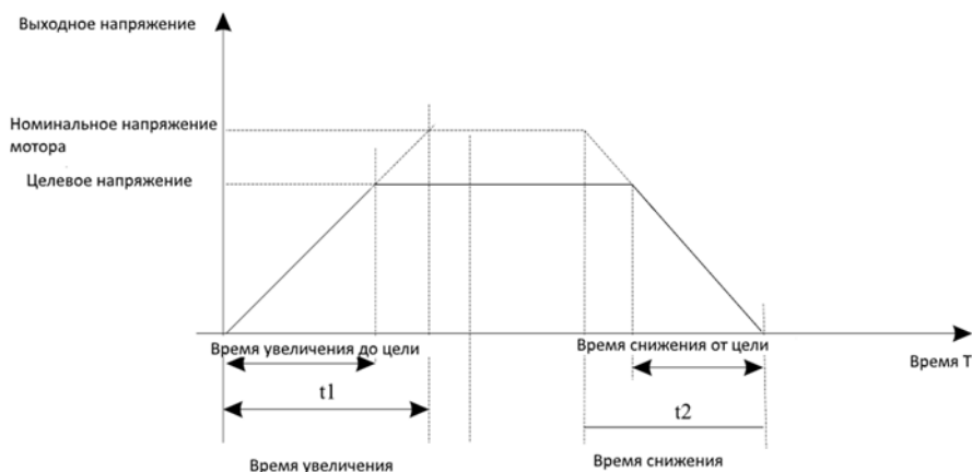
Диаграмма 5-32 Напряжение разделения V / F
