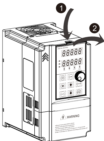
Рис. 3-3 Удаление панели управления (клавиатуры) Рис. 3-4 Установка панели управления (клавиатуры)
