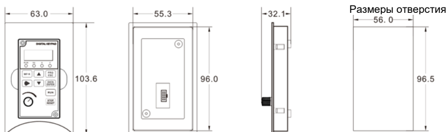
Рис 2-8 Внешний вид и размеры съемной панели у преобразователей малой мощности
