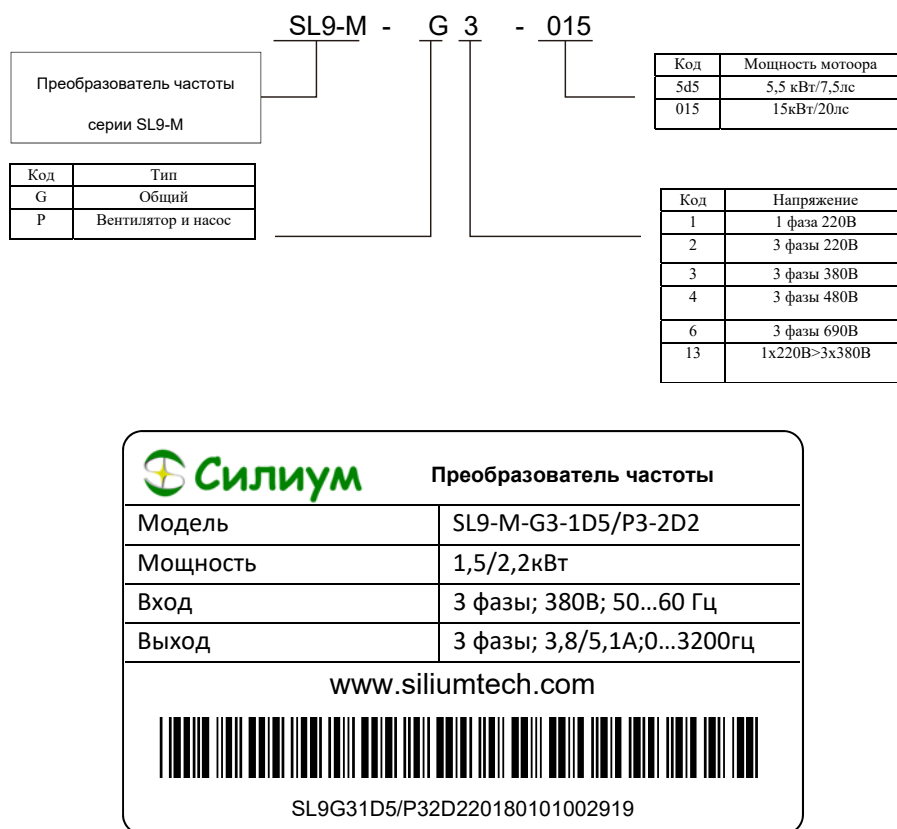
Рис 2-1 Обозначение и этикетка
