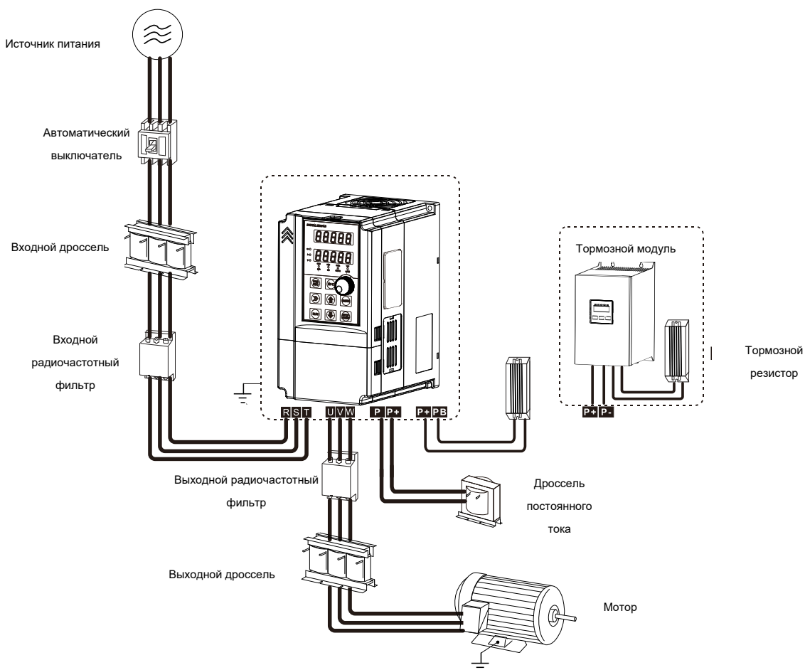
Рис. 3-2 Периферийное оборудование
