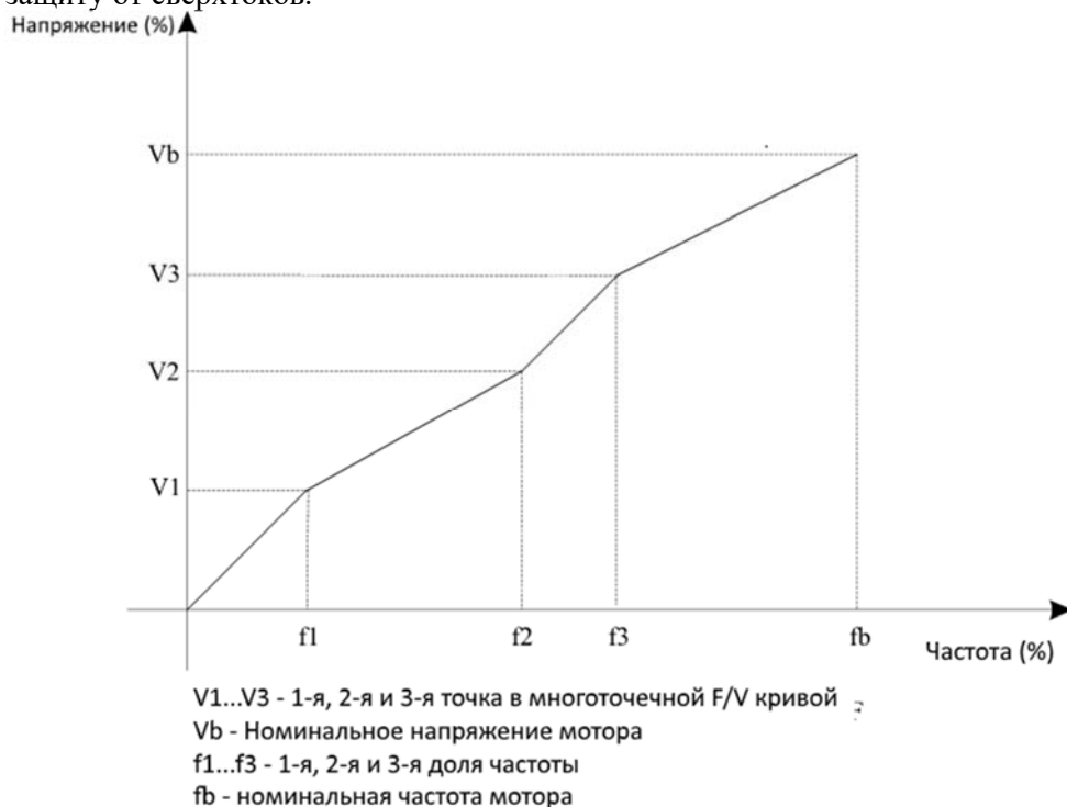
Диаграмма 5-31 Настройка многооточечной кривой V / F
