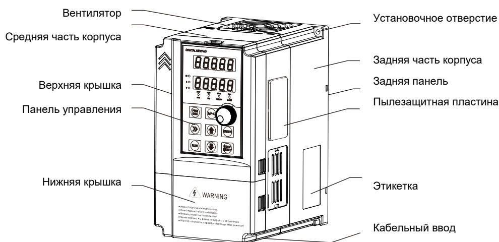
Рис 2-2 Внешний вид
