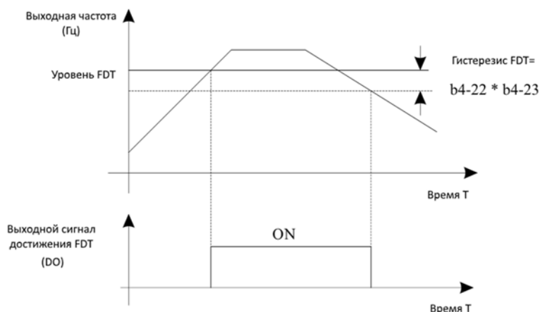
Рис. 5-14 уровень FDT
