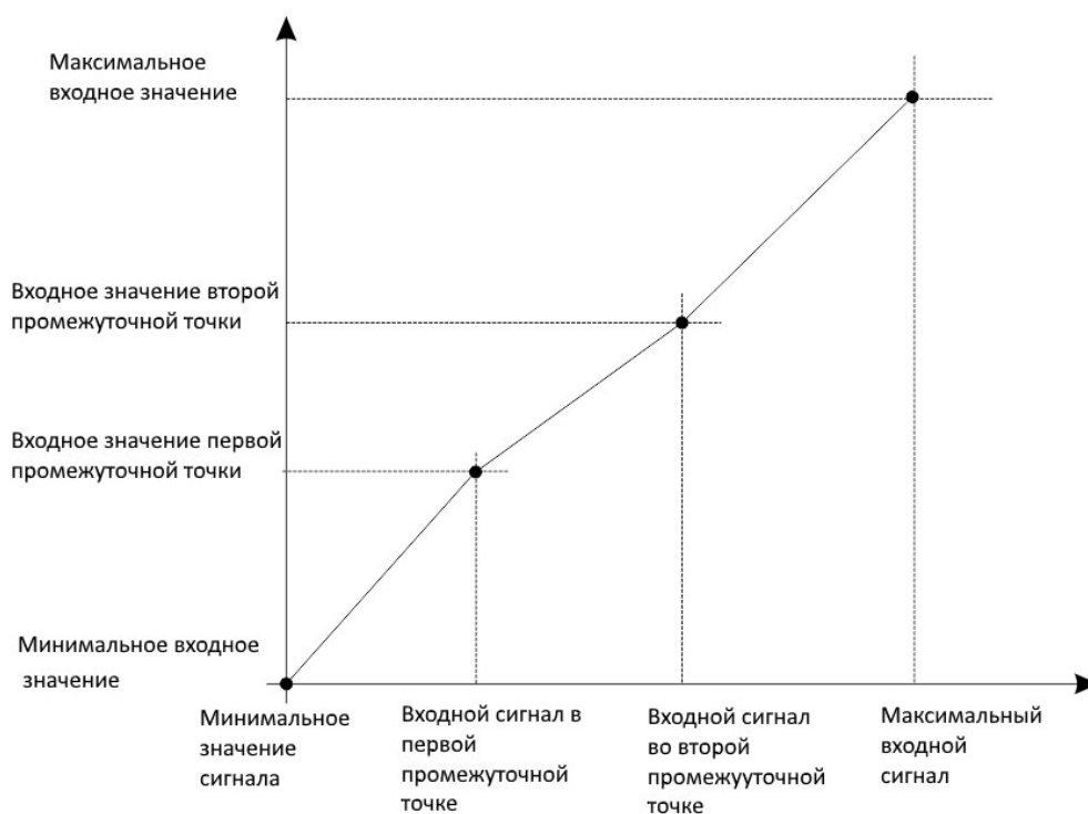
Рис. 5-21 Отношение между уровнем аналогового сигнала и входным значением
