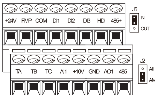
Рис 3-12 Преобразователи вход 1х220, выход 3х0...220В, 0.75~1.5кВт
