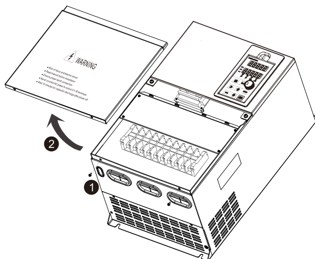
Рис. 3-6 SL9 в металлическом корпусе
