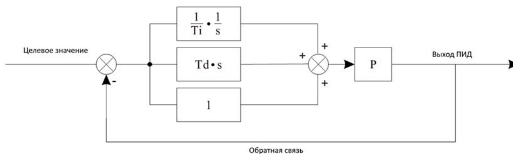
Рис. 5-25 Блок-схема ПИД-регулятора.
